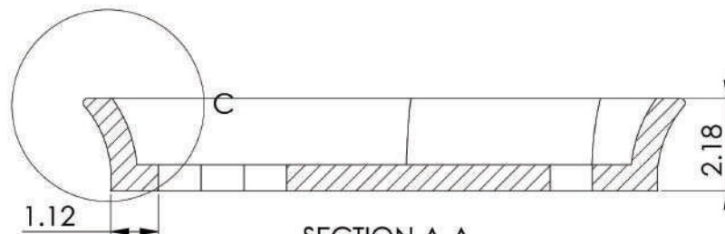
SECTION A-A SCALE 15 : 1.2
